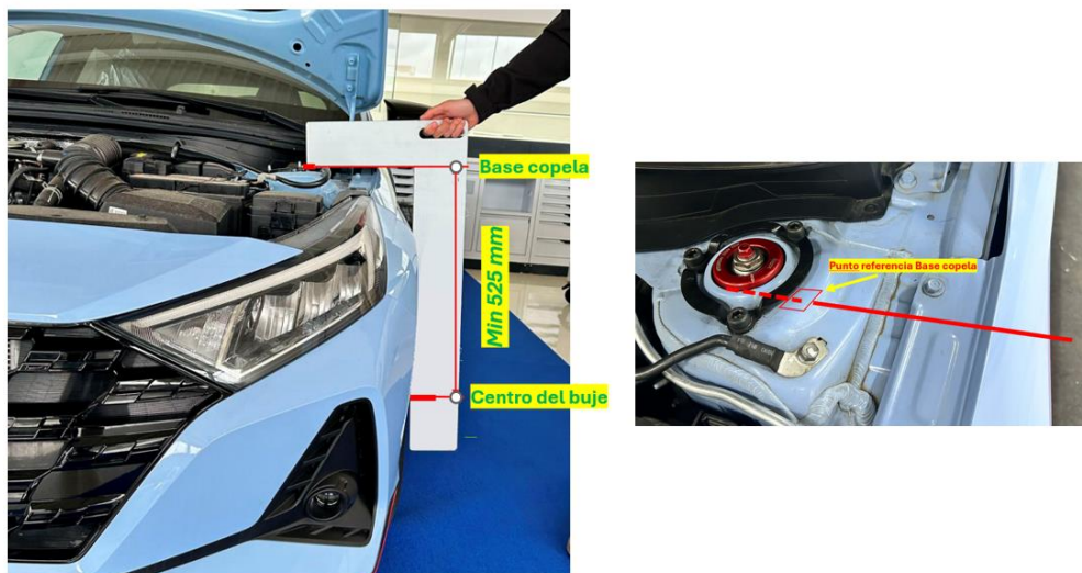
Medidas eje delantero
