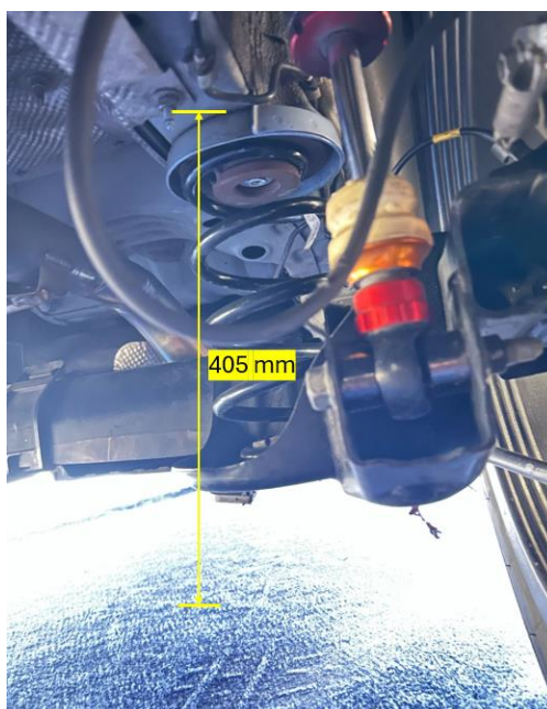
Medidas eje trasero
