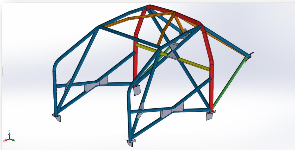
Esquema Técnico – Estructura de Seguridad Copa i20N Rallye
