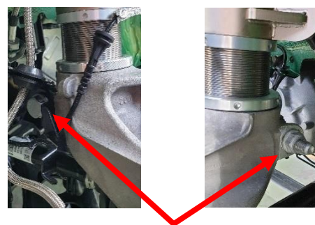
Tornillo y tuerca a aflojar para extraer el amortiguador
