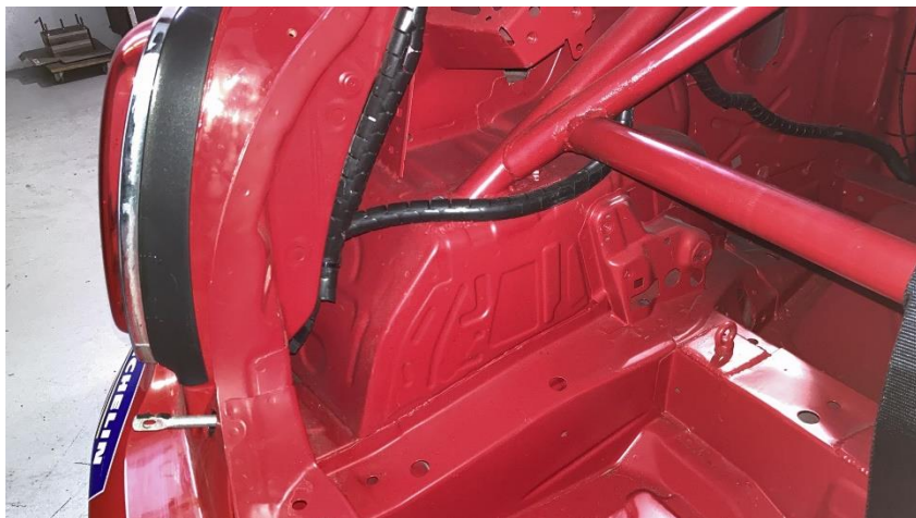
Cableado en la zona trasera izquierda
