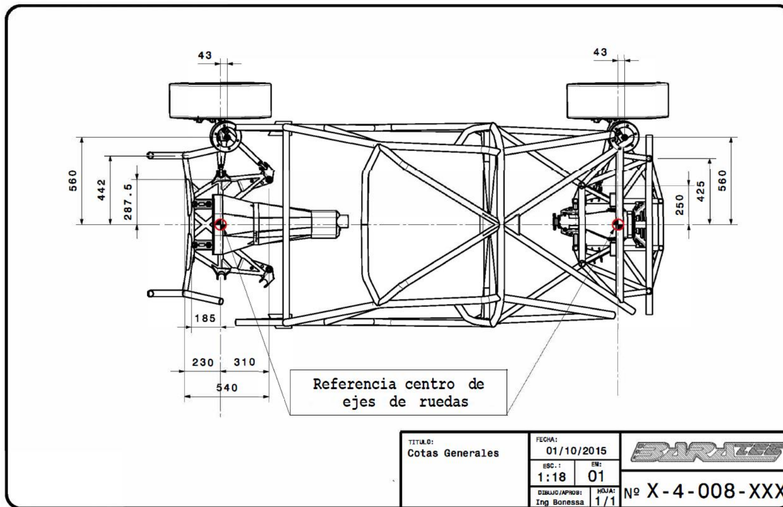
DIBUJO TÉCNICO Nº 4
