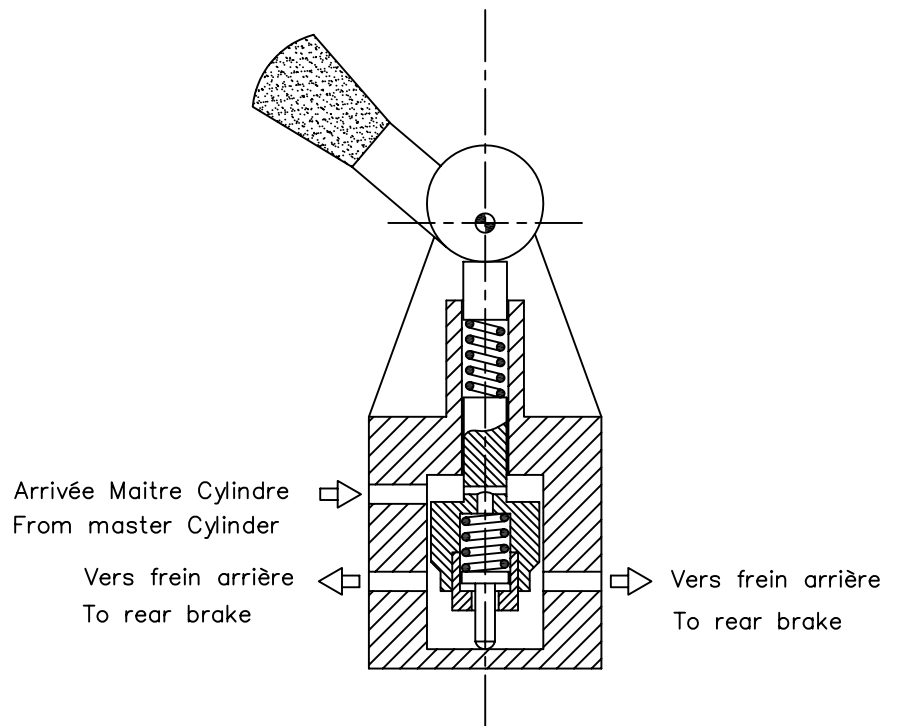
Dessin/Drawing N°263-9
