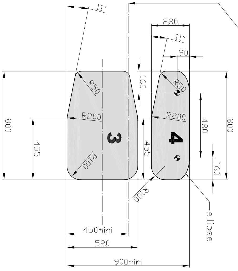
Axe longitudinale voiture Car's longitudinal centreline
