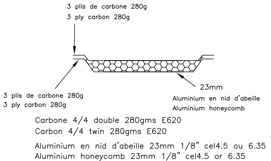
Dessin/Drawing 255-14
