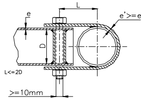
L doit être minimum La largeur de la patte doit être d'au moins 25mm L must be minimum The clamp width must be at least 25mm
